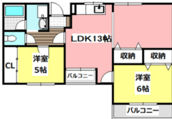
間取り写真
