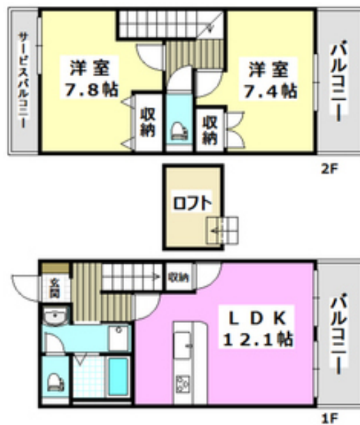
▲間取写真
