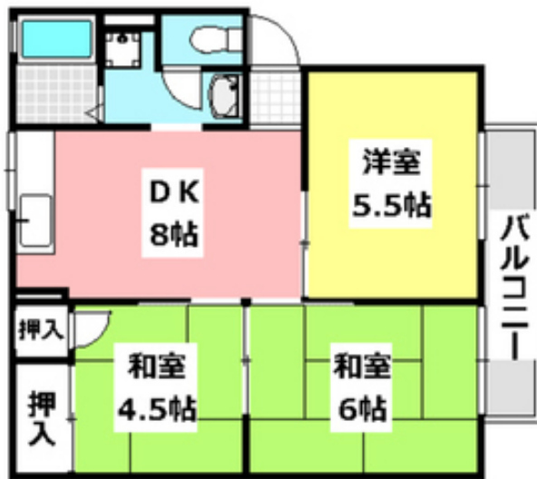
▲間取写真
