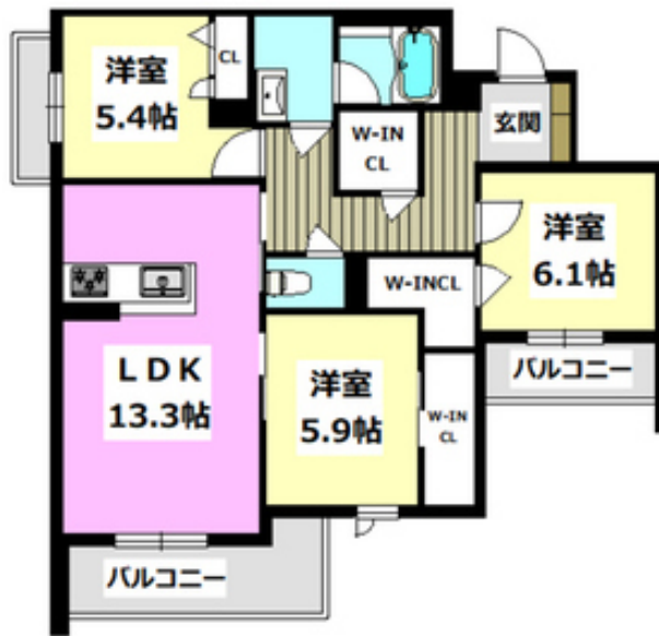
間取写真
