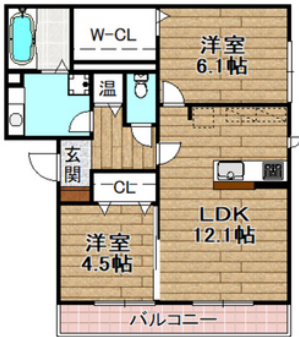
▲間取写真
